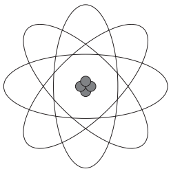
Sommerfeld
