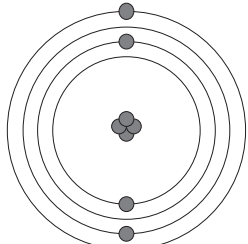
Rutherford-Bohr
